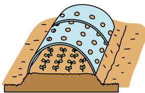
図3 トンネルの被覆
